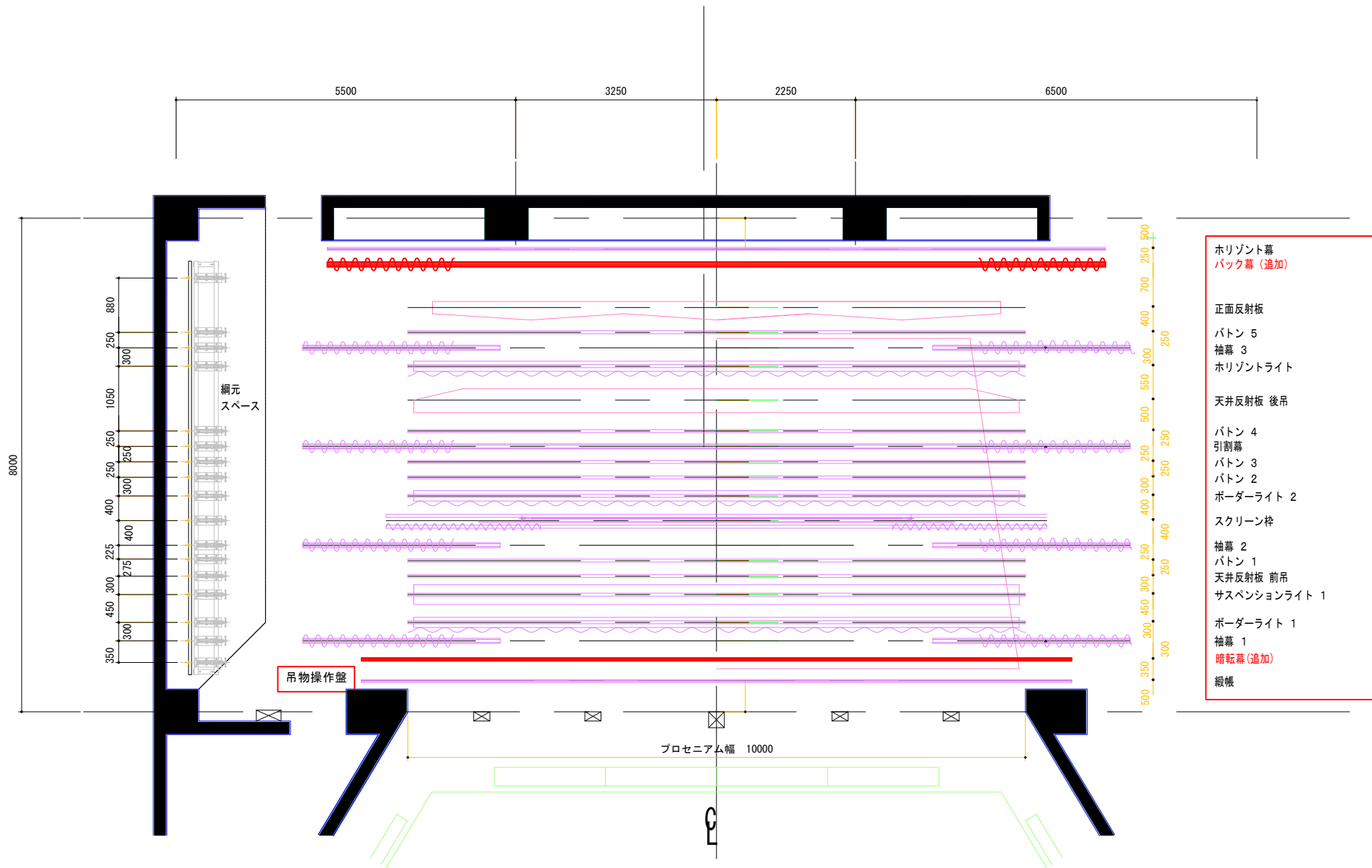
吊り物配置図(小ホール)
